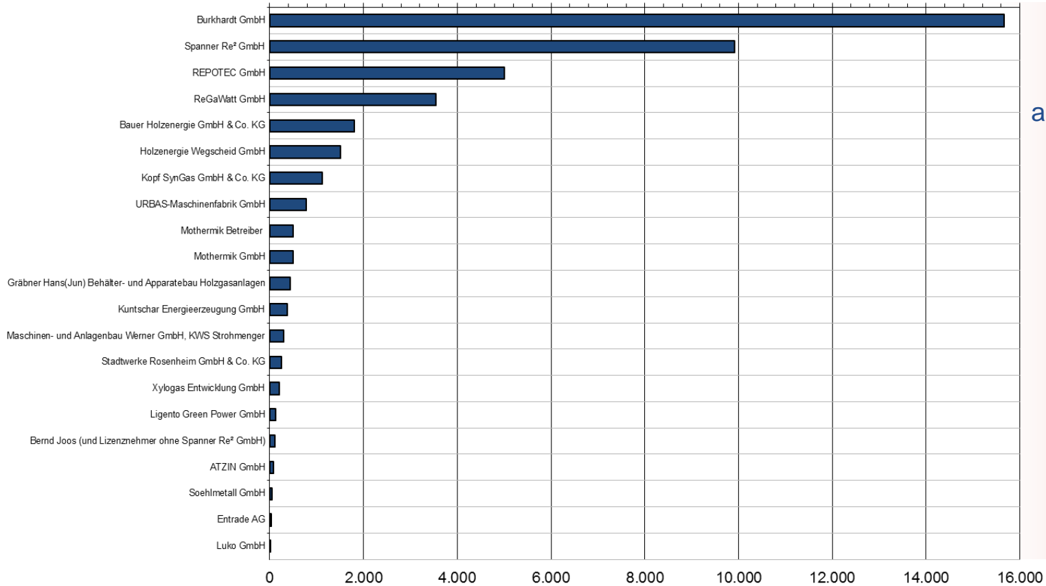
elektrische Gesamtleistung P_{el} in kW (Deutschland)
